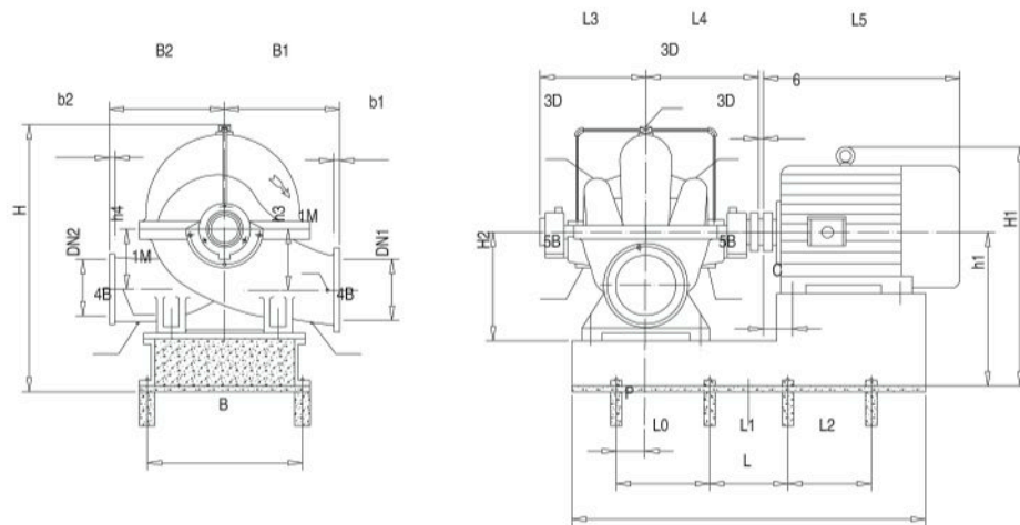
连接螺纹尺寸 Connect nut size
