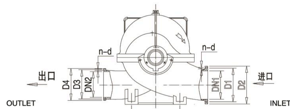
法兰尺寸图
